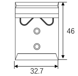
DIN Rail Clip
